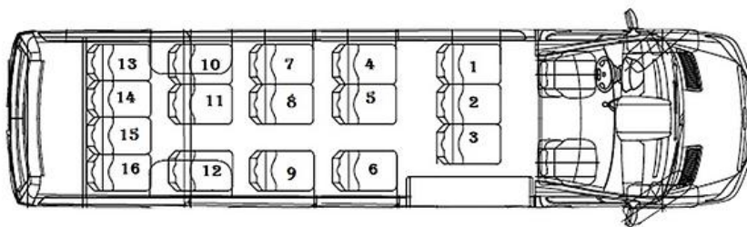
Схема мест в автобусе
